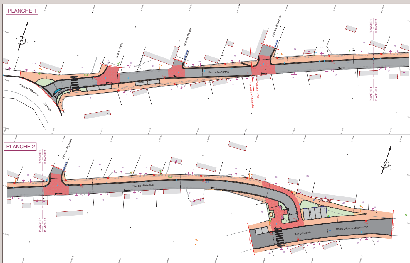
Plan d'aménagement de la rue de Marienthal
